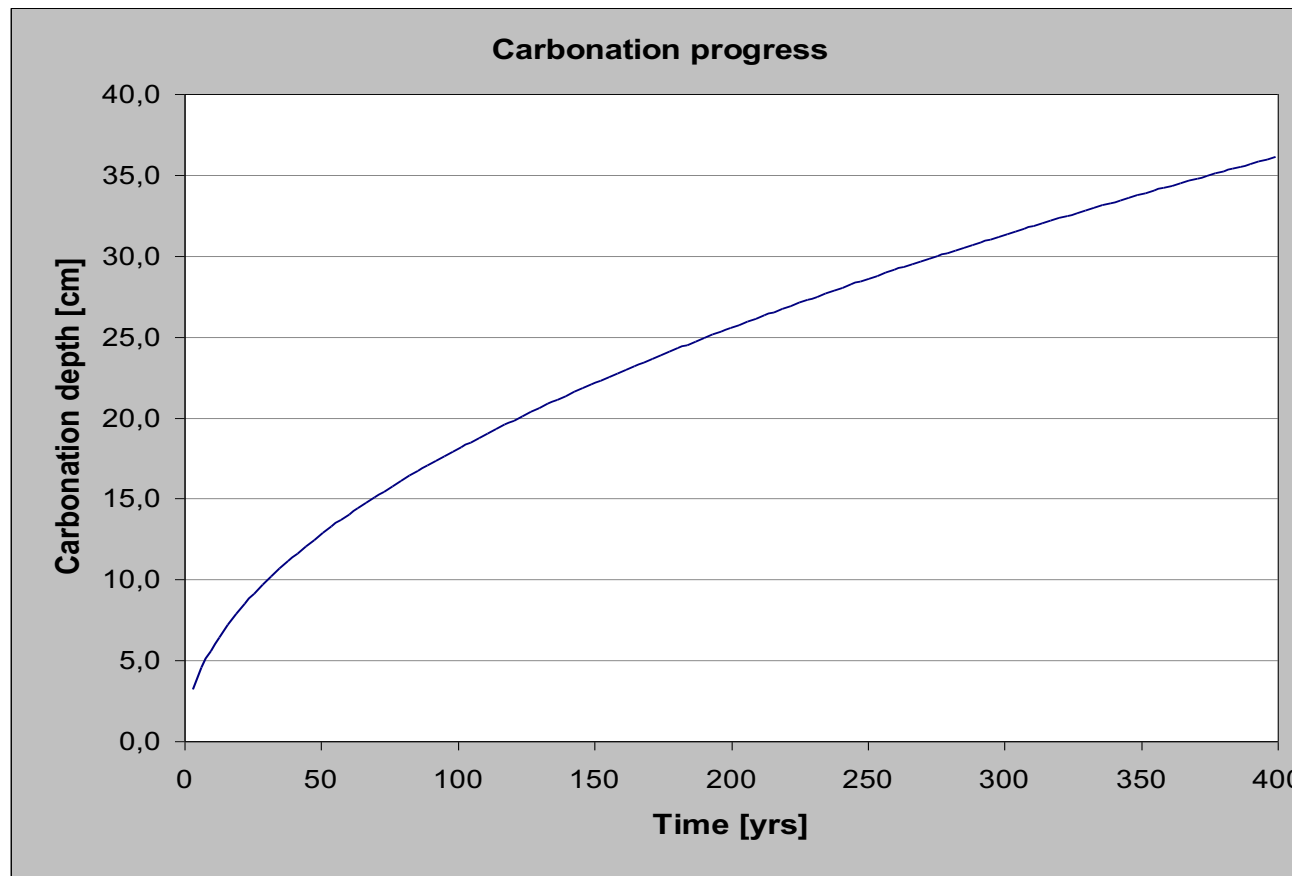
Carbonatation des mortiers à la chaux
